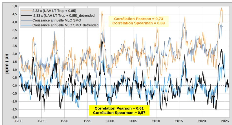
Figure 5c : Comparaison après ajustement (courbe orange) via sensibilité a = 2,33 (corrélation post ajustement = 0,73 ou 0,69). Comparaison entre séries 'detrended' → corrélation = 0,61 ou 0,57 .
