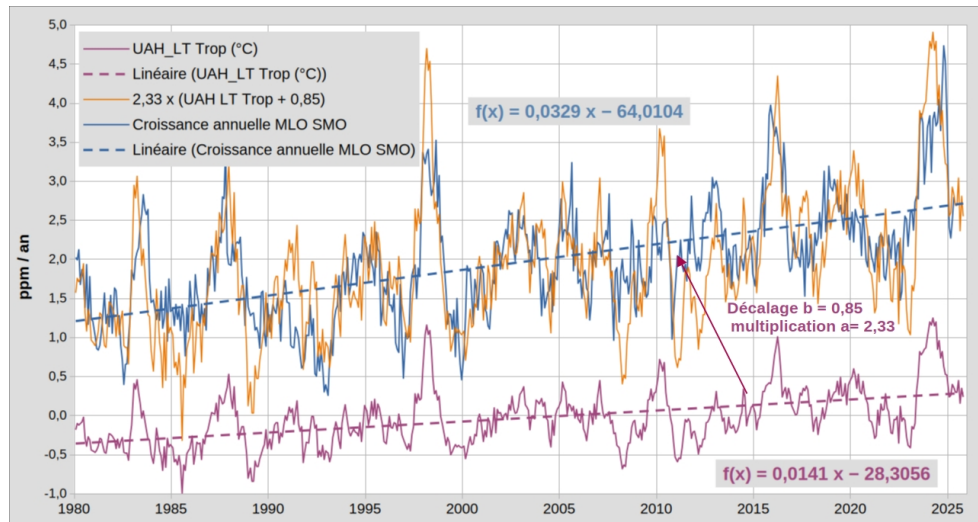
Figure 5b : Croissance annuelle du CO 2 atmosphérique (moyenne MLO SMO) et anomalie UAH_LT_Tropics (courbe violette). Ajustement UAH_LT_Tropics (courbe orange) via le rapport des 2 tendances = sensibilité a = 0,0329 / 0,0141 = 2,33 .
